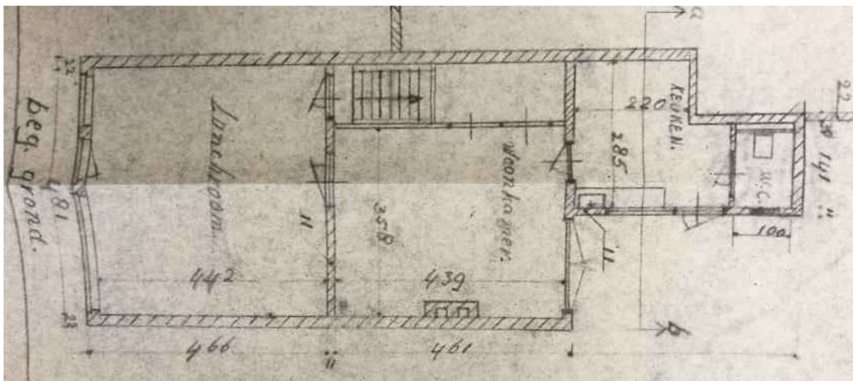
Figuur 46: De bestaande toestand van de begane grond zoals deze in 1960 werd getekend, is vermoedelijk de negentiende-eeuwse situatie. De voorgevel is links.
