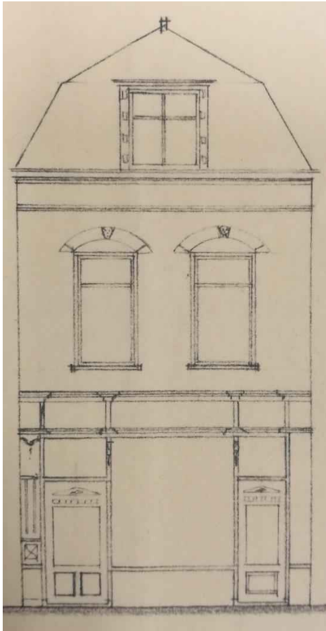
Figuur 36: Tekening van de gevel die rond het midden van de negentiende eeuw werd opgetrokken. Detail uit een bouwtekening uit 1966, toen onder meer de dakkapel werd gewijzigd.
