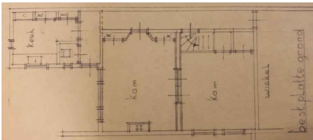
Figuur 70: De bestaande, vermoedelijk negentiende-eeuwse, indeling op de verbouwingsplattegrond van 1963.
