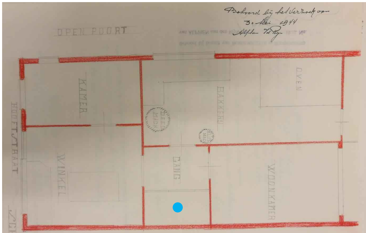
Figuur 32: Bouwtekening uit 1944. De gang met de trap naar de bovenwoning is niet meer aanwezig. De blauwe stip markeert de vermoede locatie van de trap in deze tijd. Straatzijde: links.
