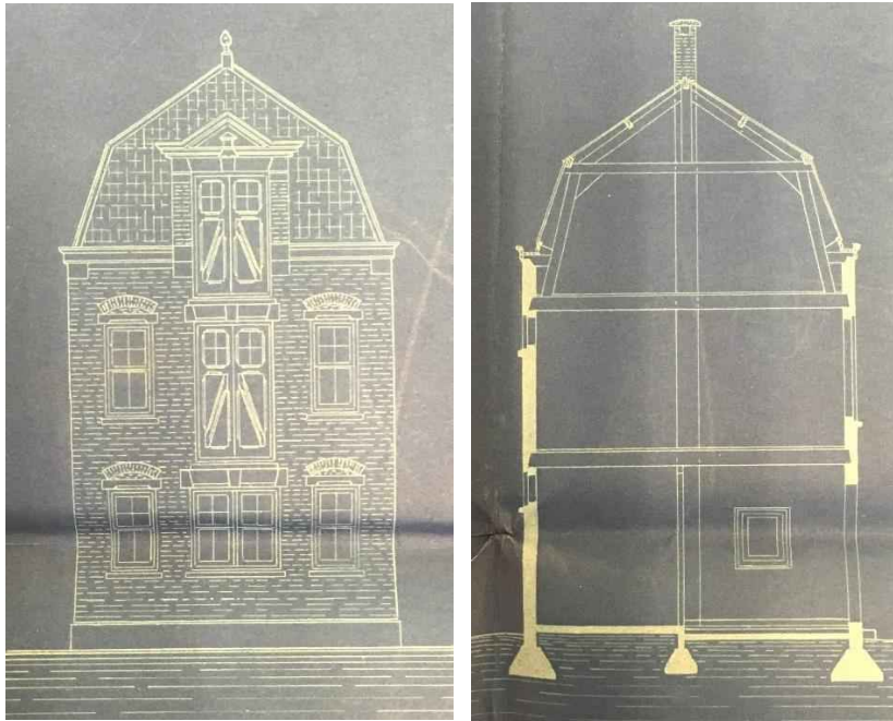
Figuur 54: Links het ontwerp van de voorgevel, rechts de doorsnede van de nieuwbouw.
