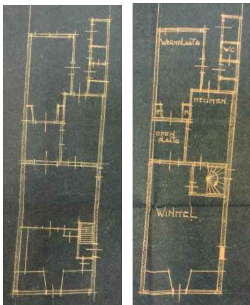
Figuur 51: Links de bestaande toestand in 1928, rechts de gewijzigde.
