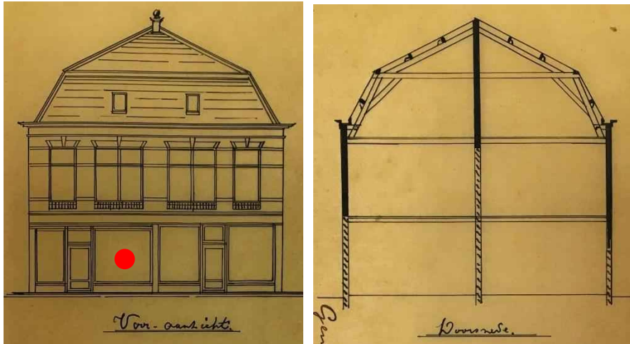
Figuur 45: Het voorgevelfront en de doorsnede van Hooftstraat 55-57 op een de bouwtekening uit 1905. Op de doorsnede is goed zichtbaar dat bestaand muur werk (gearceerd) bij deze nieuwbouw behouden bleef. De rode stip markeert nummer 55.
