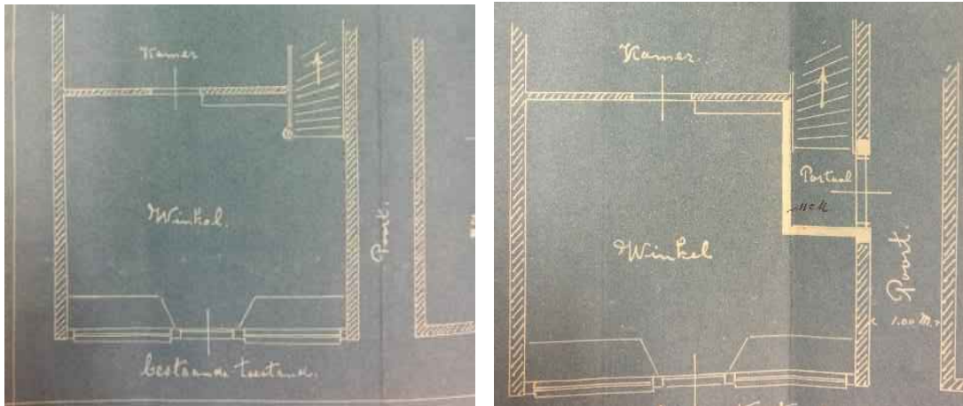
Figuur 50: Detail uit een bouwtekening die in 1923 werd ingediend. Het betreft de destijds bestaande, hoogstwaarschijnlijk nog negentiende-eeuwse, situatie. Rechts, de gewijzigde toestand waarbij een afzonderlijke entree naar de bovenwoning werd gerealiseerd
