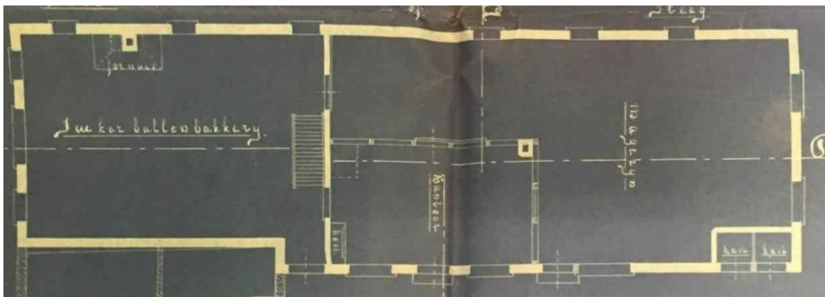
Figuur 56: Indeling van de begane grond van de nieuwbouw in 1931. De voorgevel ligt links.
