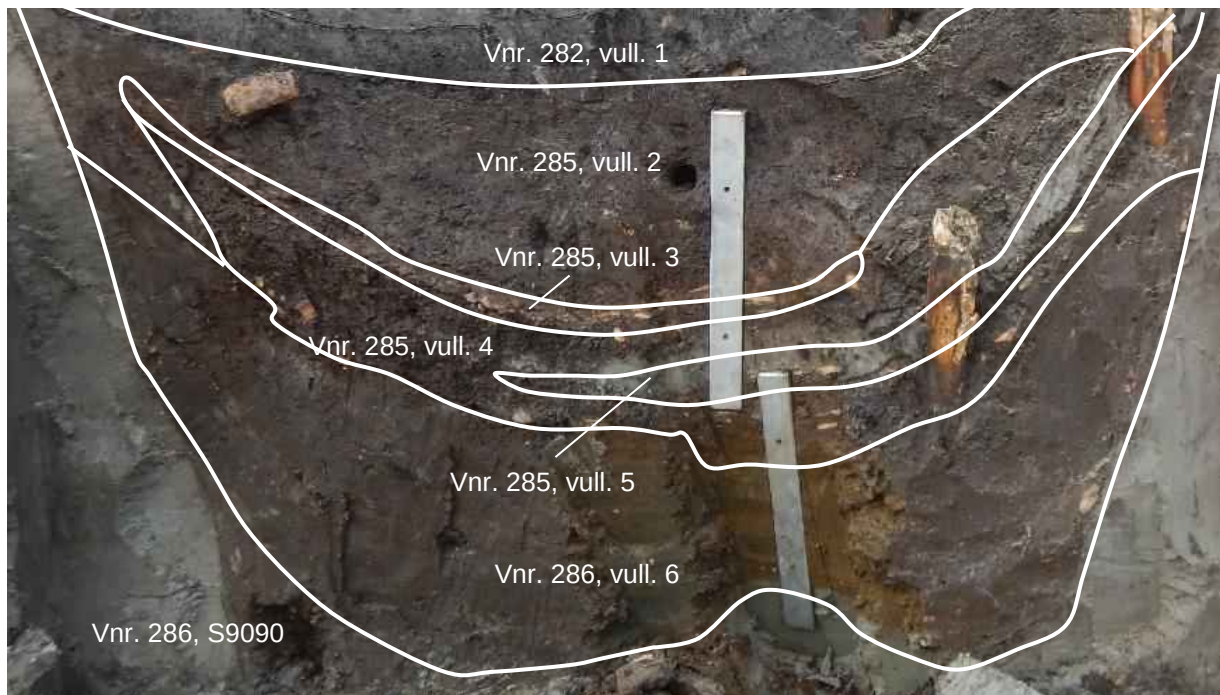
Figuur 114: Overzicht van de onderzochte lagen voor de kwalitatieve palynologische analyse.
