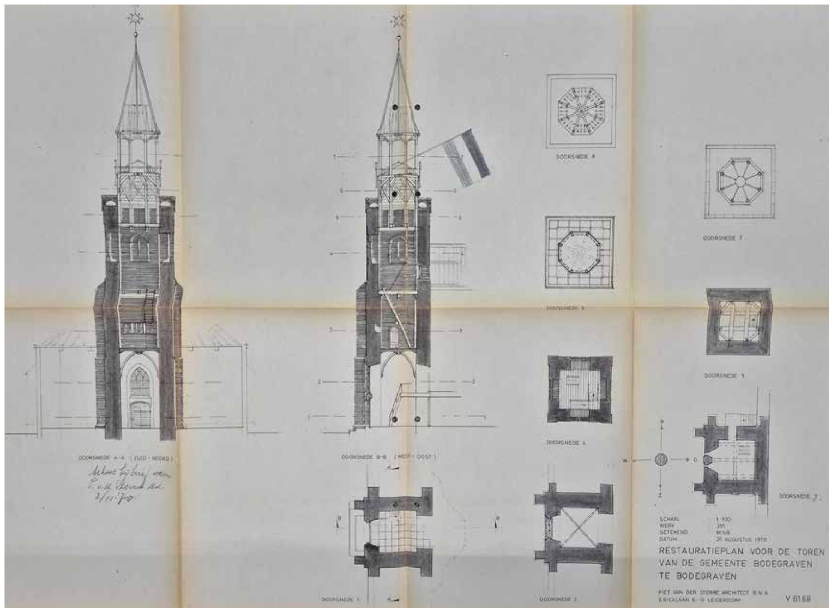
afbeelding 241. Doorsneden en plattegronden toren: Restauratieplan voor de kerktoeren, 20 augustus 1970, door Piet van der Sterre. Bron: RHCVV, toegang B051, inv.nr.: 810.
