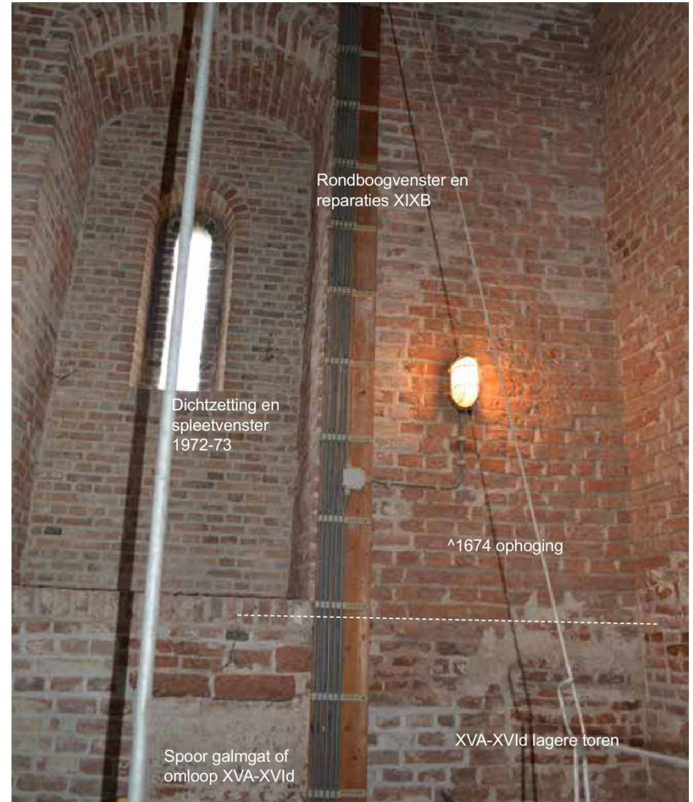
afbeelding 62. Zicht richting het venster in de noordgevel van de derde geleding van de toren. De grotere segmentboogvormige opening werd in dichtgemetseld (1972-73) en voorzien van een spleetvenster met ronde bovenzijde (1972-73).
