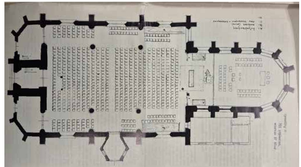
afbeelding 237. Plattegronden van twee varianten voor een nieuwe interieuropstelling in de Dorpskerk door architect Van der Sterre (1968-1971). De variant opstelling II, werd uiteindelijk doorgevoerd en is tot op heden zo aanwezig. Bron: RHCVV, toegang B058a, inv.nr.: 75.
