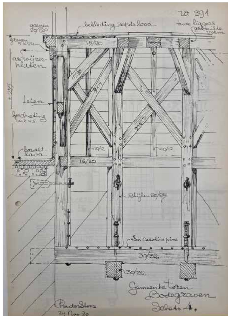
afbeelding 244. Schetsen restauratieplan kerktoeren, augustus 1970, door Piet van der Sterre. Blad 4 en 5. Bron: RHCVV, toegang B051, inv.nr.: 810.
