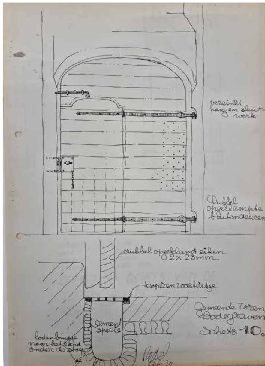
afbeelding 247. Schetsen restauratieplan kerktoeren, februari 1970 en januari 1972, door Piet van der Sterre. Blad 10 en 11. Bron: RHCVV, toegang B051, inv.nr.: 810.
