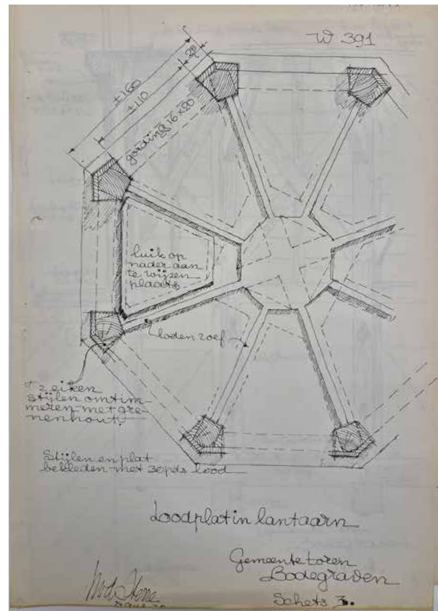
afbeelding 243. Schetsen restauratieplan kerktoeren, augustus 1970, door Piet van der Sterre. Blad 1 en 3. Bron: RHCVV, toegang B051, inv.nr.: 810.
