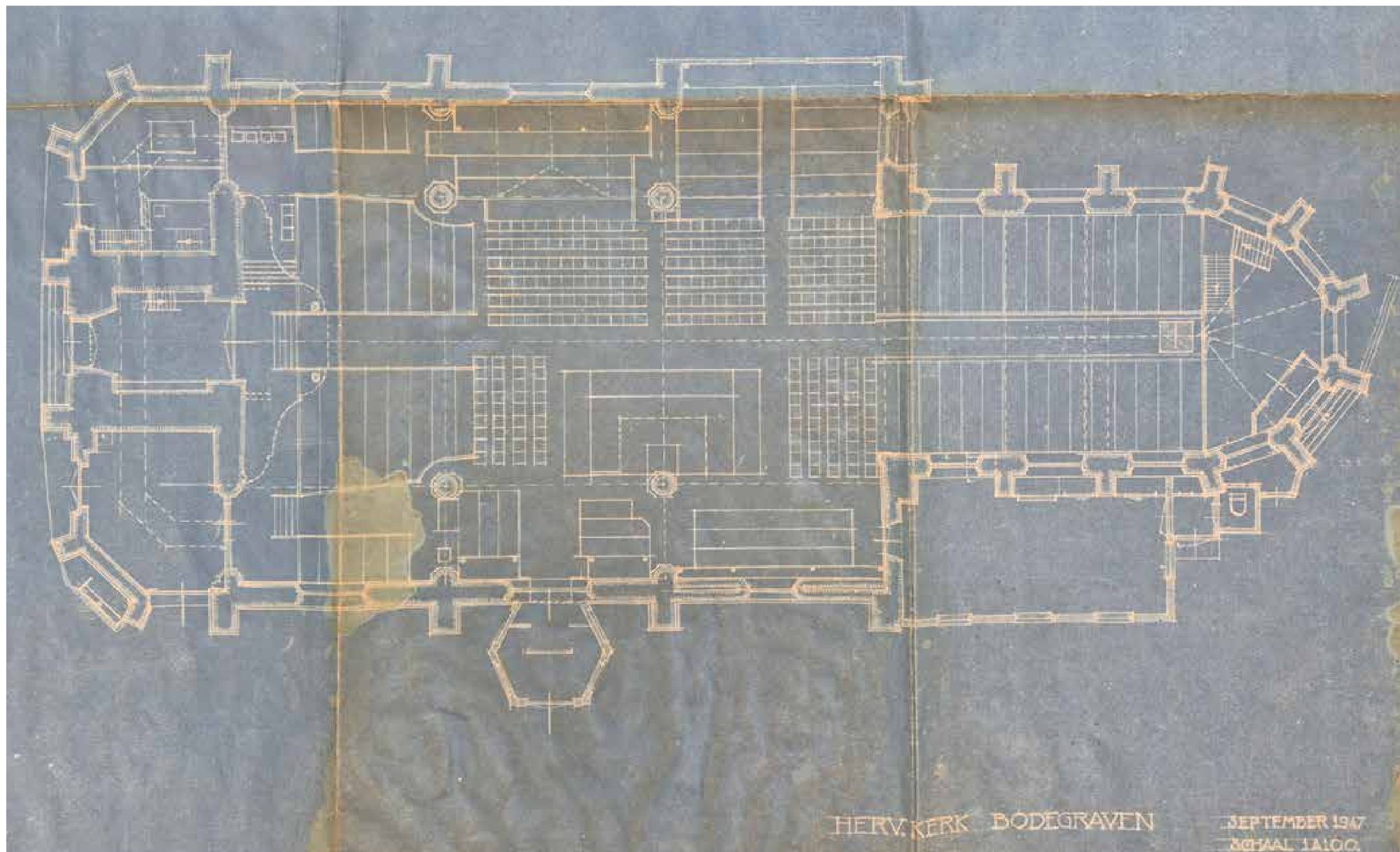
afbeelding 228. Plattegrond uit september 1947 van de bestaande toestand, vermoedelijk opgesteld door architect J.P.L. Petri. Bron: RHCVV, toegang B058a, inv.nr.: 95.
