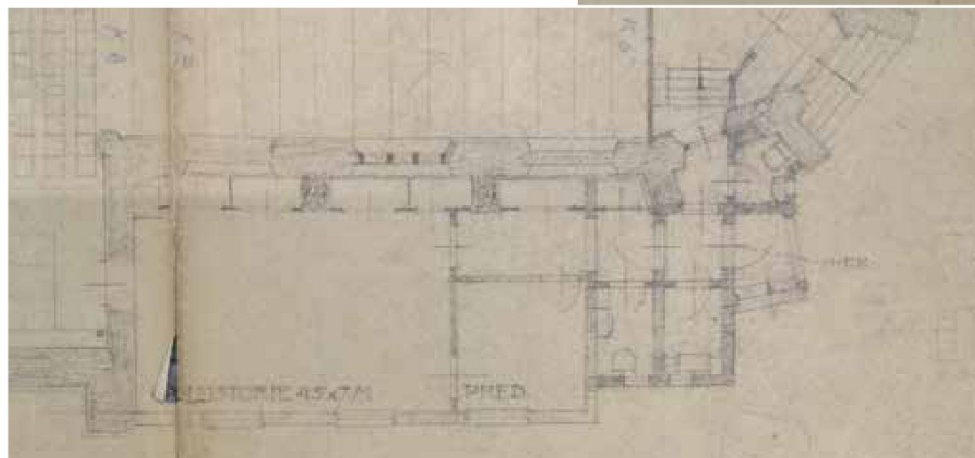
afbeelding 230. Plattegrond uit juli 1948 van de nieuwe toestand, vermoedelijk opgesteld door architect Petri, voor de uitbreiding van het kerkgebouw en verbouwing van de consistorie (zie linksonder). De aanbouw aan de noordzijde werd niet gerealiseerd! Bron: RHCVV, toegang B058a, inv.nr.: 95.
