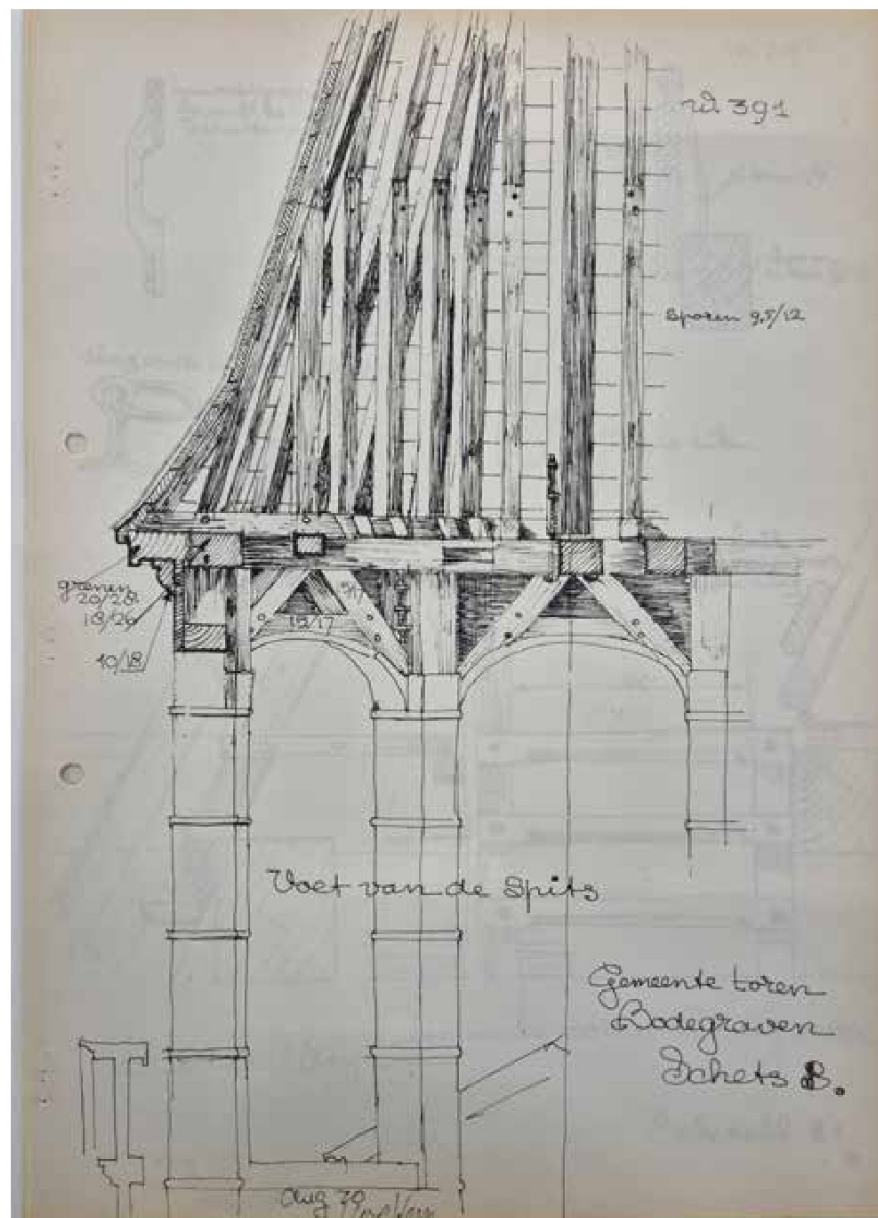
afbeelding 246. Schetsen restauratieplan kerktoeren, augustus 1970, door Piet van der Sterre. Blad 8 en 9. Bron: RHCVV, toegang B051, inv.nr.: 810.
