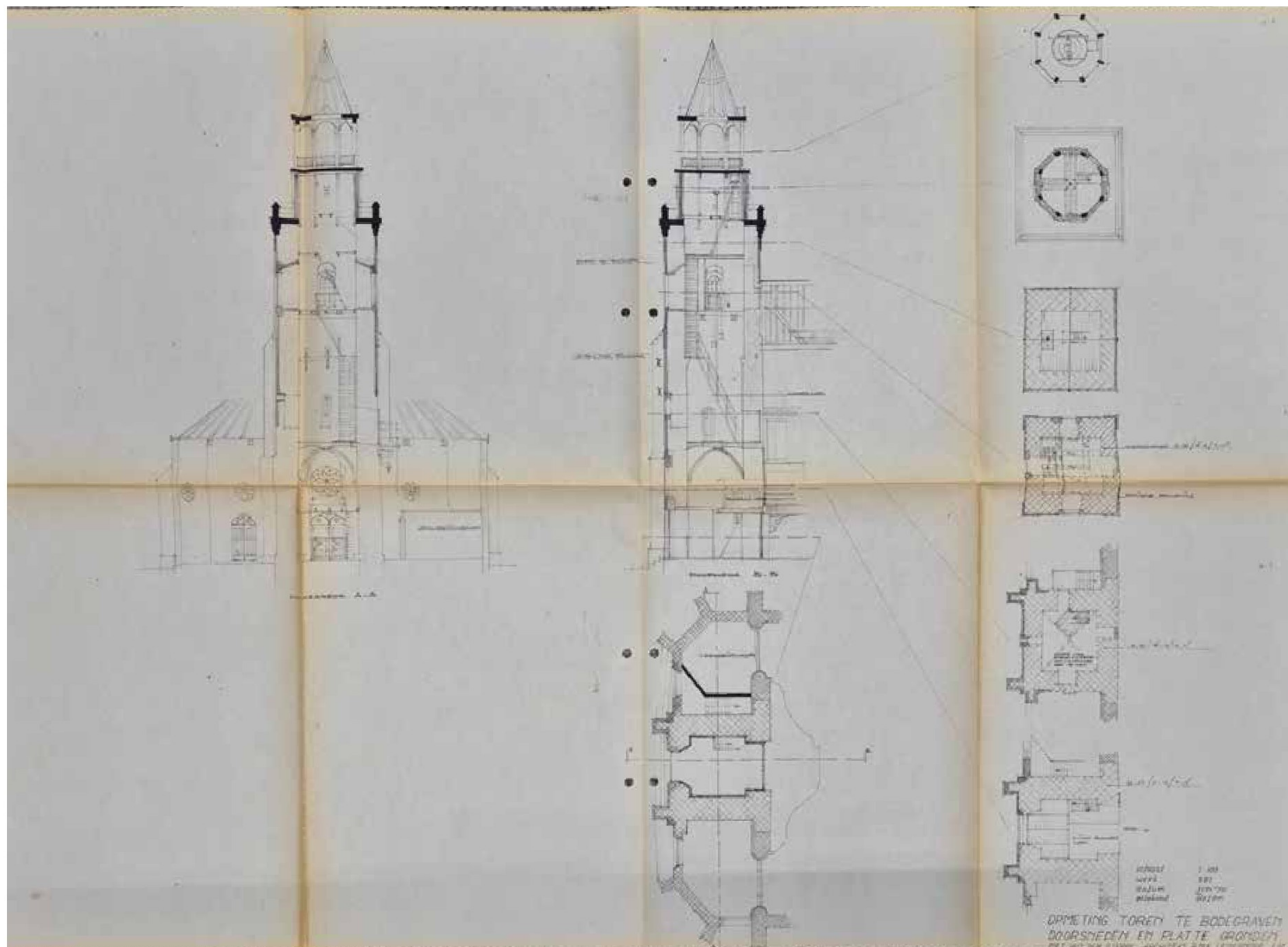
afbeelding 239. Opmetingstekeningen doorsneden en plattegronden van de bestaande toestand van de toren t.b.v. restauratieplan voor de kerktoeren, juni 1970, door Piet van der Sterre. Bron: RHCVV, toegang B051, inv.nr.: 810.
