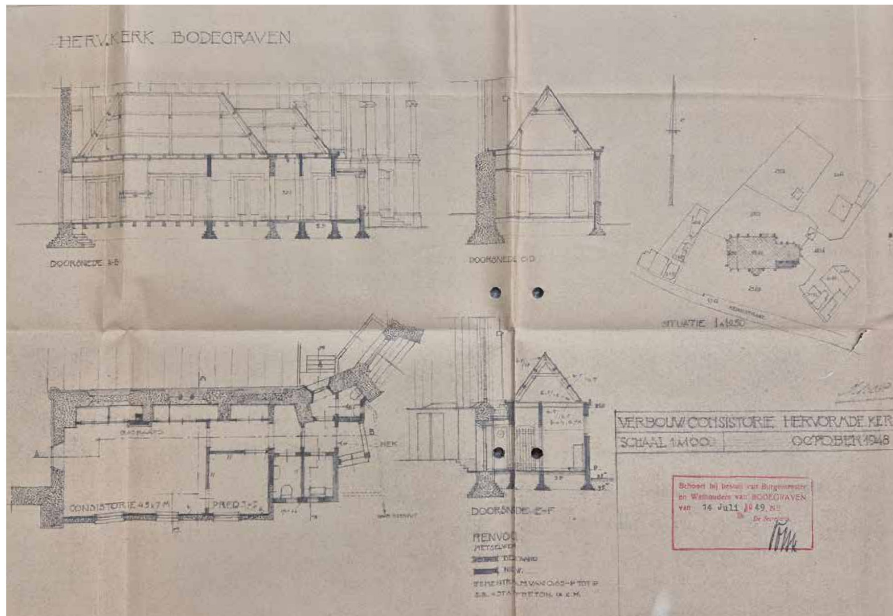
afbeelding 231. Plattegrond en doorsneden voor de verbouwing en uitbreiding van de consistorie door architect J.P.L. Petri, oktober 1948. Bron: RHCVV, toegang B057, inv. nr.: 1949-22.
