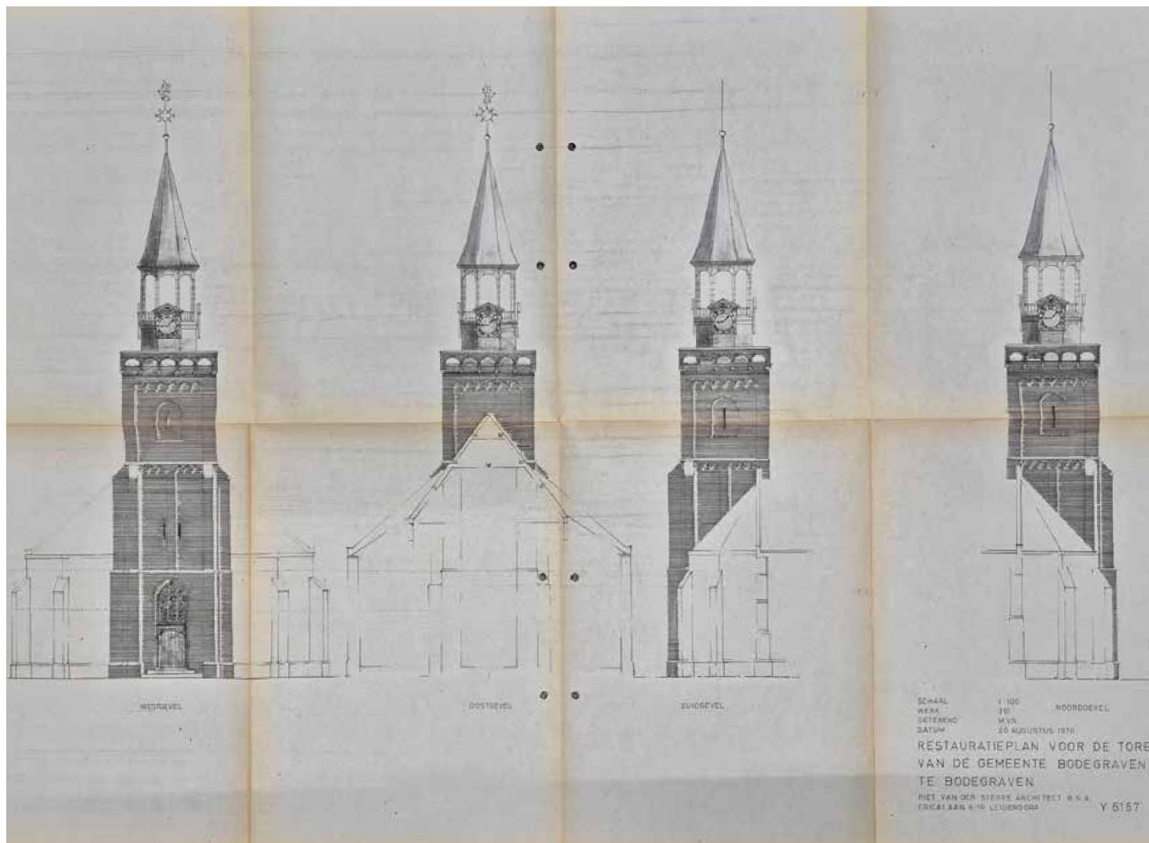
afbeelding 242. Gevelaanzichten toren: Restauratieplan voor de kerktoren, 20 augustus 1970, door Piet van der Sterre. Bron: RHCVV, toegang B051, inv.nr.: 810.
