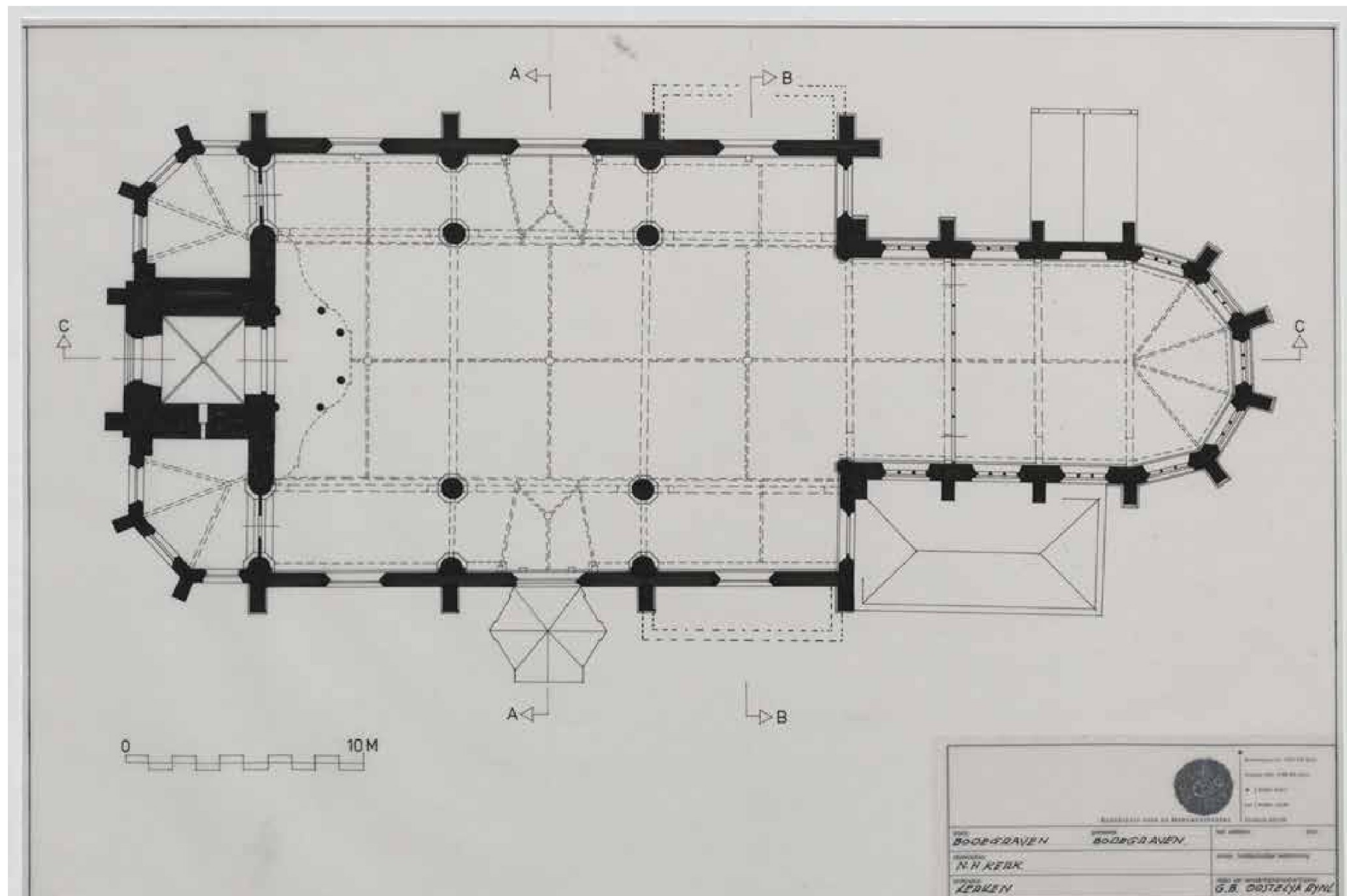
afbeelding 251. Plattegrond toestand na restauratie 1971. Door Architectenbureau van Dam- van der Sterre 1972, getekend door J.J. Jehee naar W.J. Berghuis 1999. Bron: RCE, doc.nr. BT-031320.
