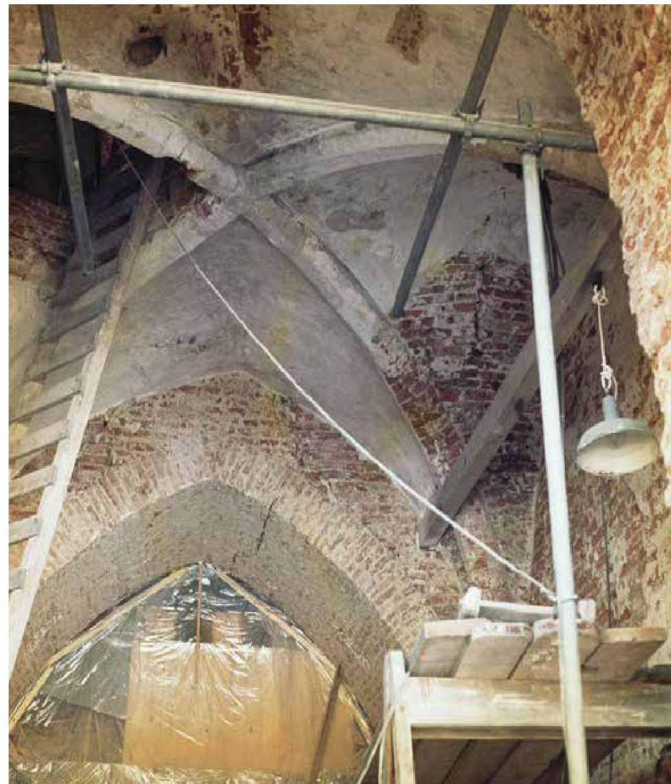
afbeelding 215. Torengewelf met opening, gedurende de restauratie, ca. 1972. Bron: RHCRL C026, inv.nr.: X3789.
