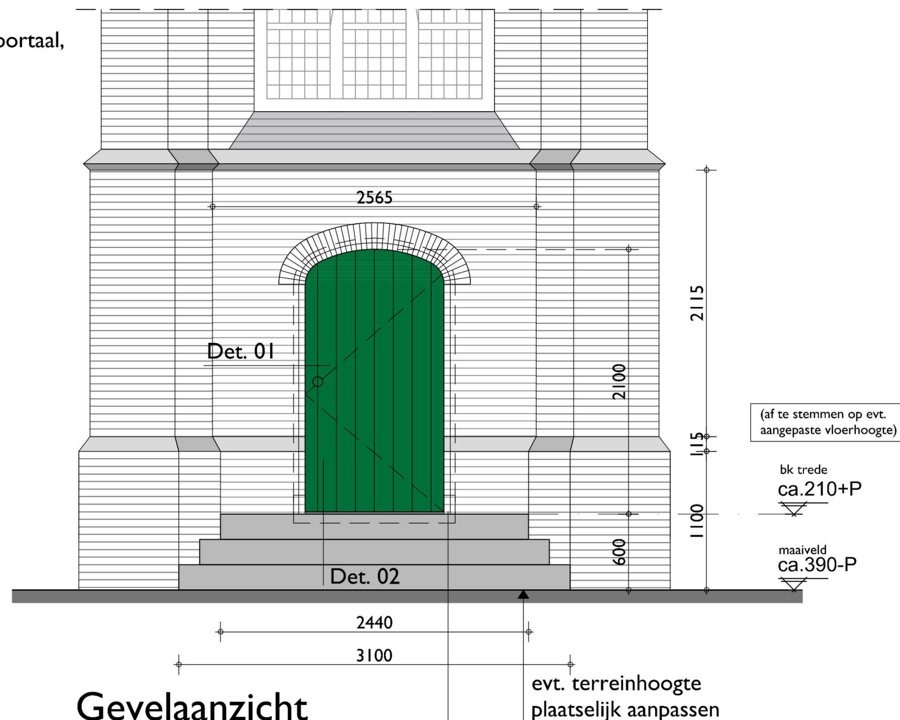
Gevelaanzicht bestaande situatie
