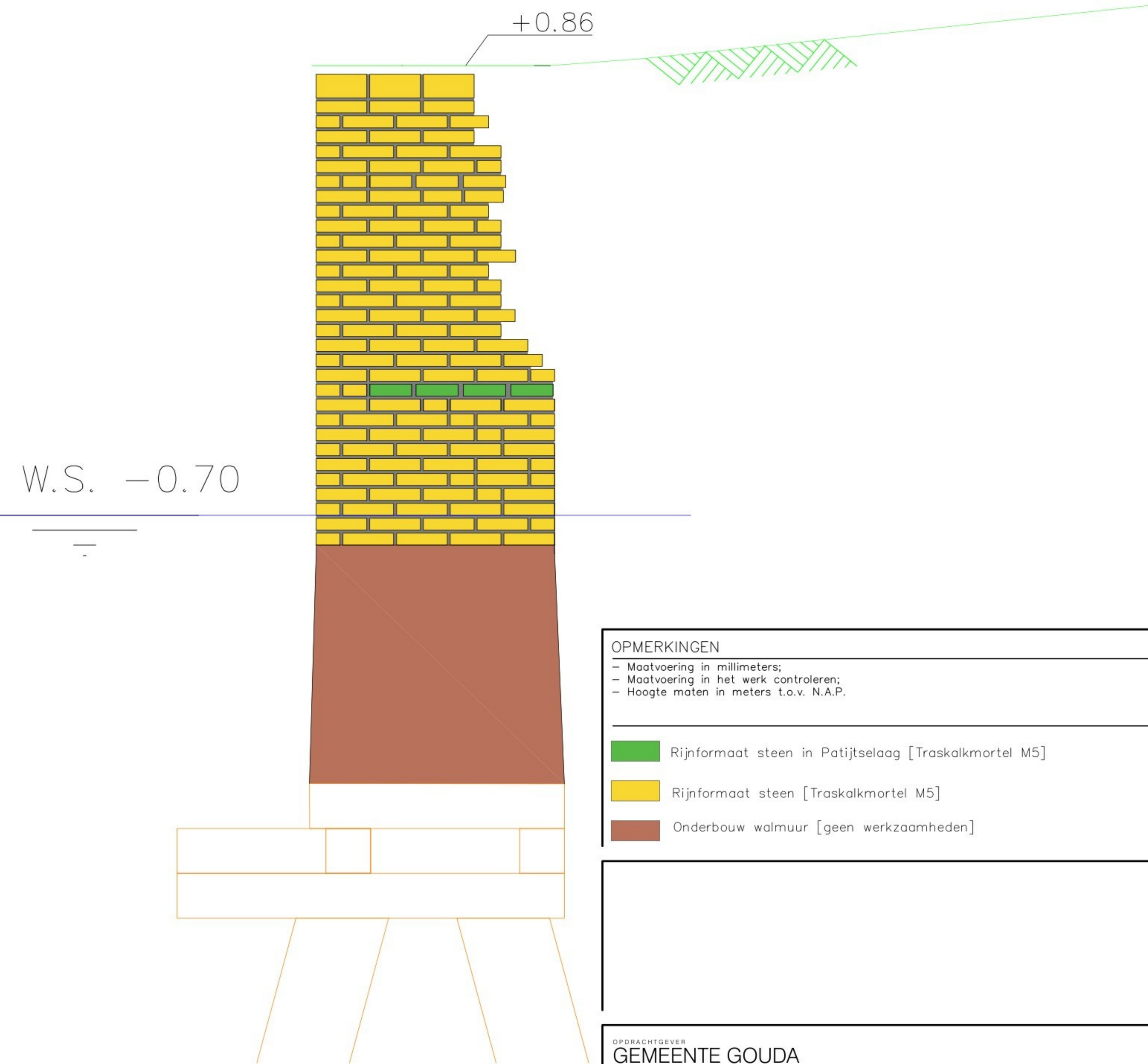
Zijaanzicht 1:10 Bestaande situatie*
