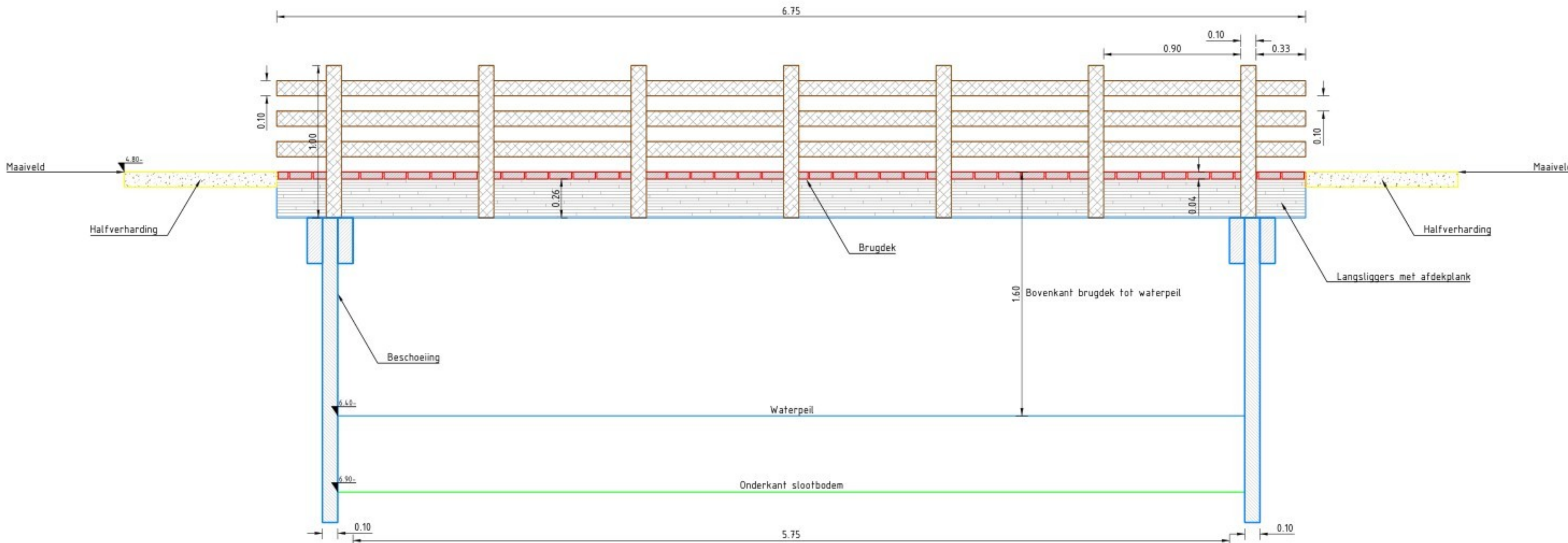
LANGSDOORSNEDE VOETGANGERSBRUG B-B schaal 1:20
