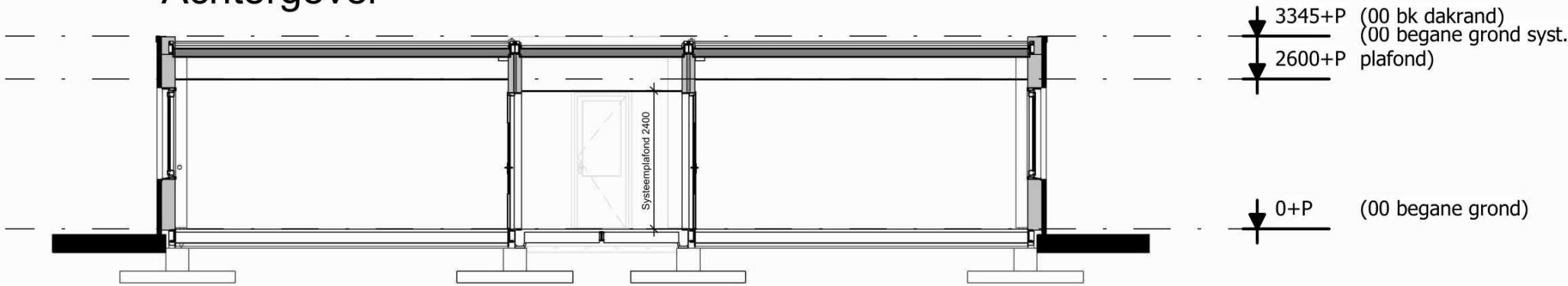
Doorsnede A-A
