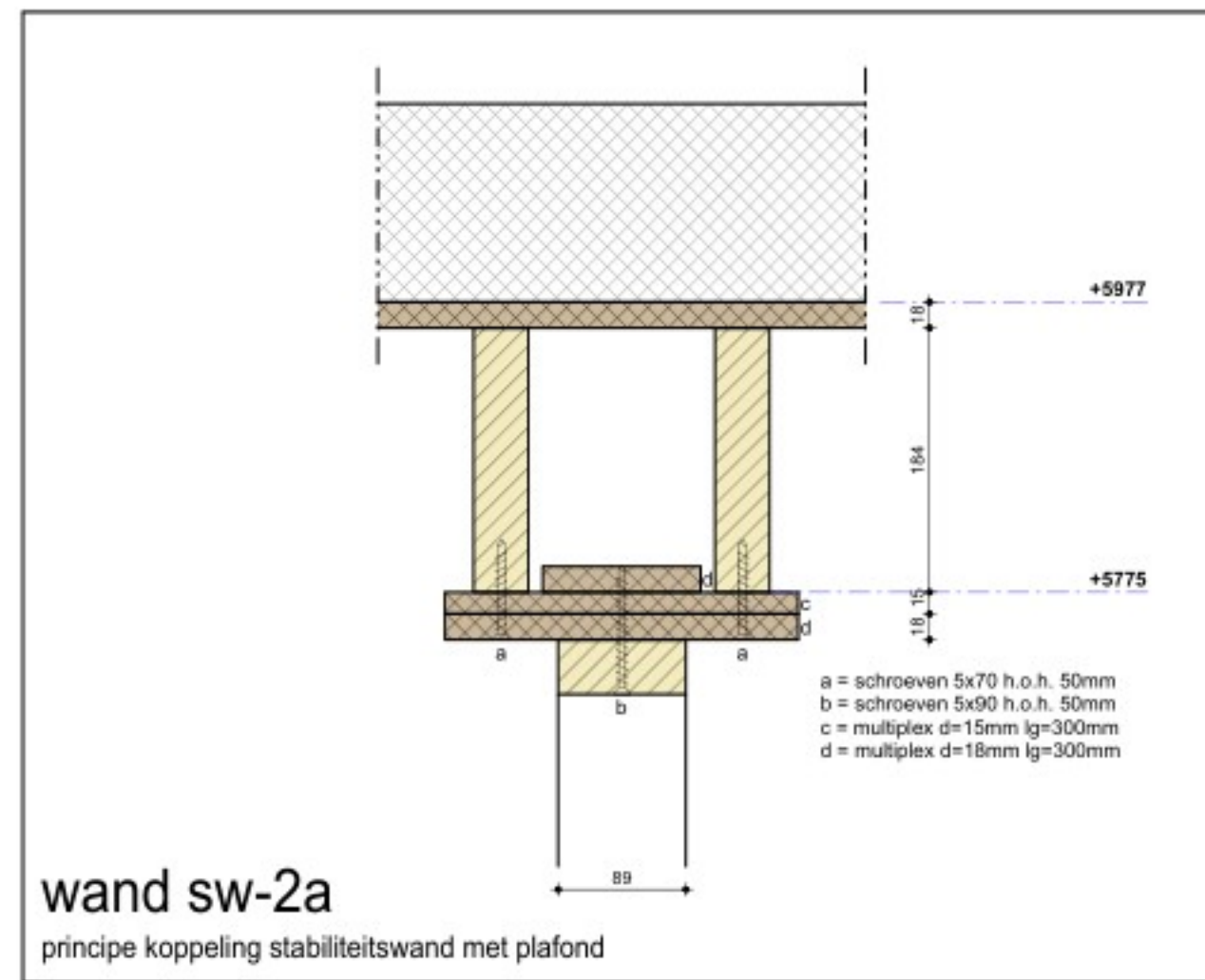
Det 101 1 : 10
