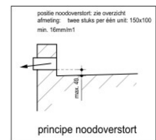
principe noodoverstort
