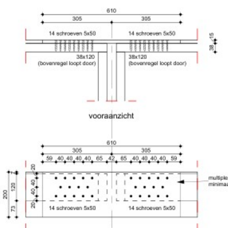
Det 101 1 : 10
