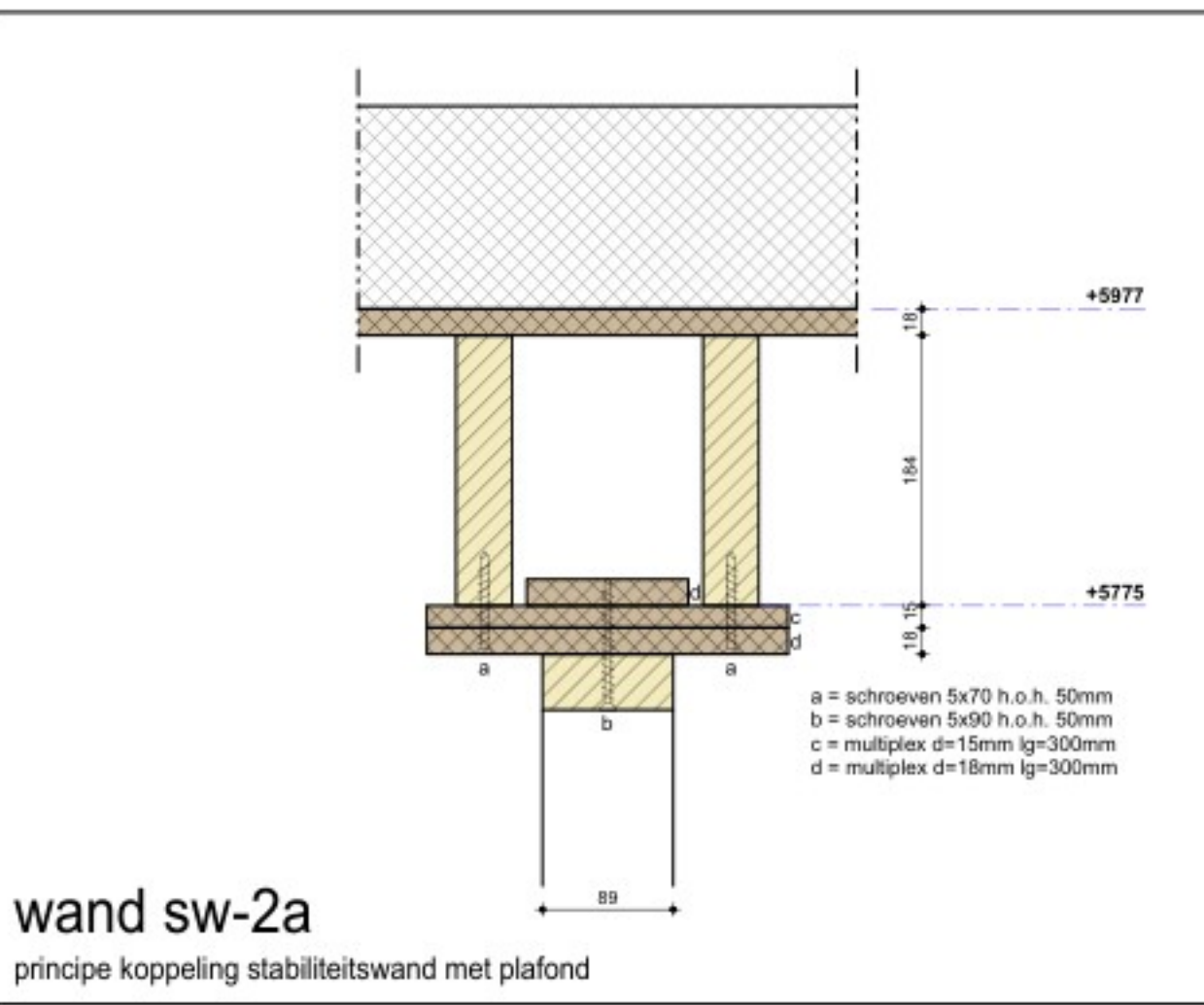
Det 101 1 : 10
