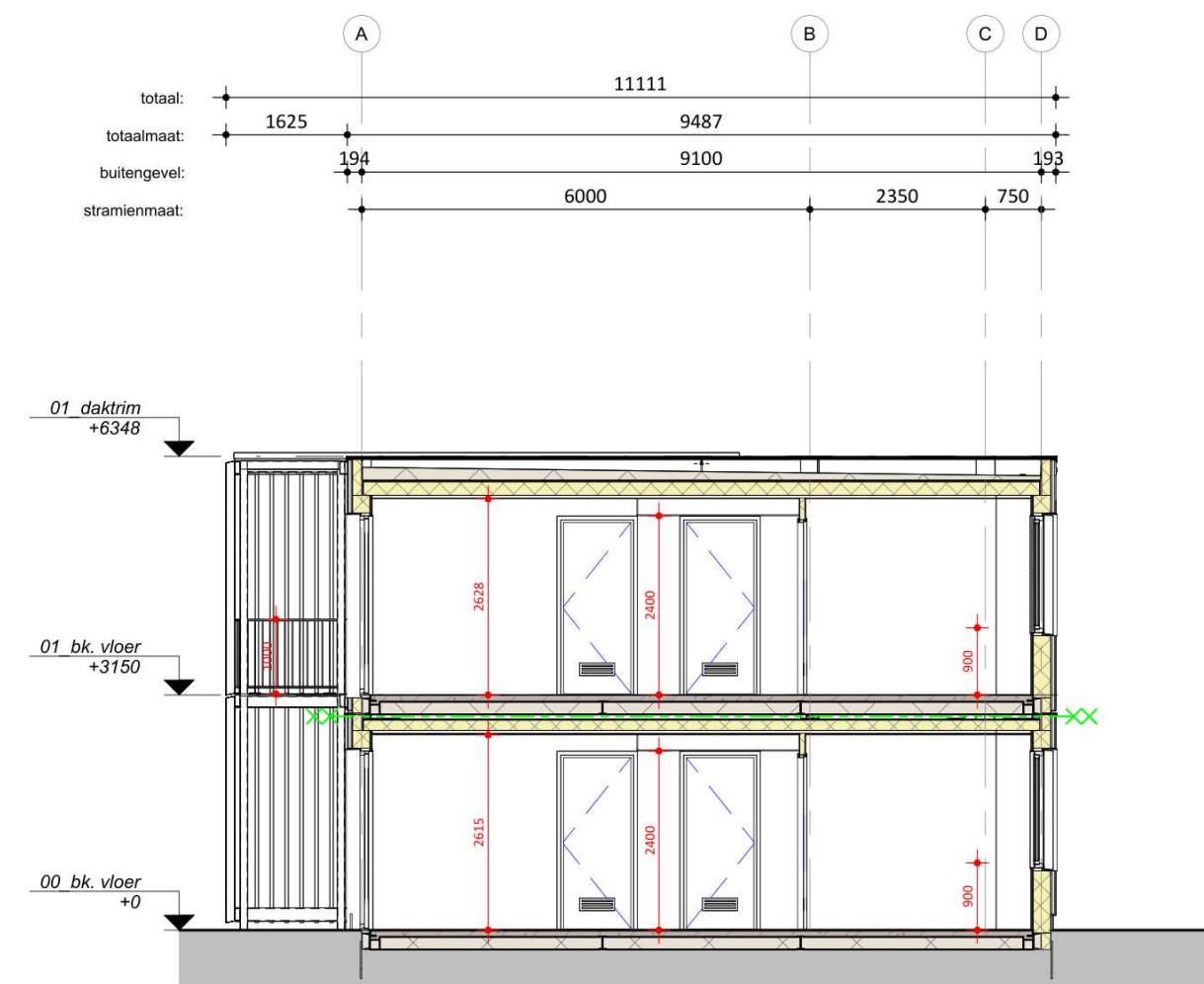
Doorsnede C
