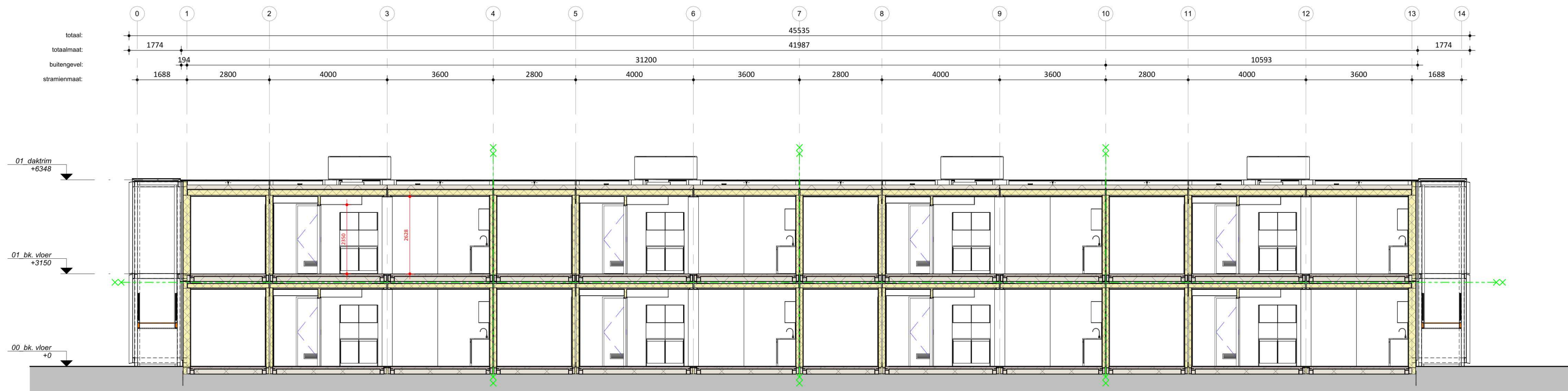
Doorsnede B
