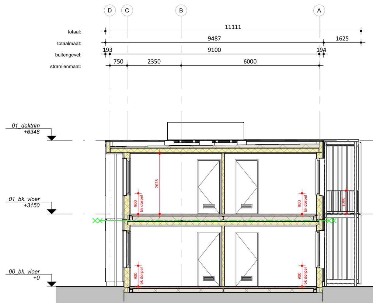
Doorsnede A
