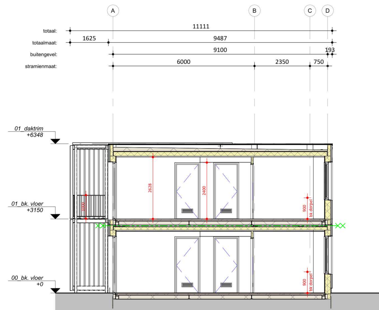
Doorsnede C
