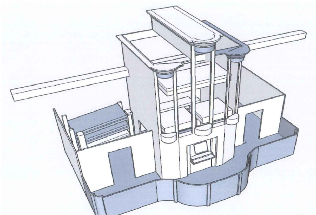
Opengewerkte tekening van de plaatsing van de blaasbalgen voor de restauratie van het Louis II Delahaye orgel in de Dorpskerk te Moordrecht
