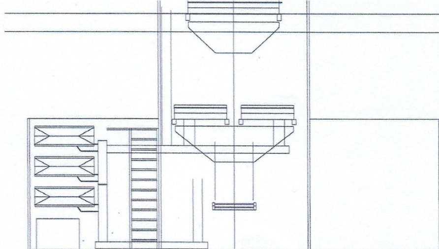
DOORSNEDE C-D
