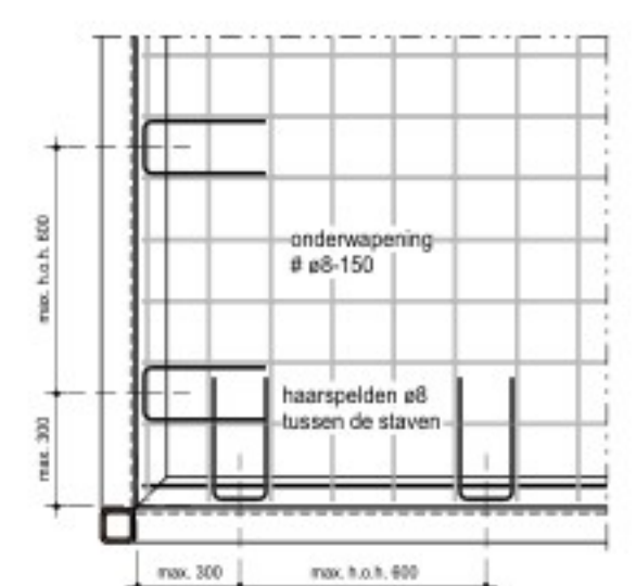
principe plaatsing van de haarspelden bij onderwapening t.p.v. bovenwapening zijn geen haarspelden nodig.
