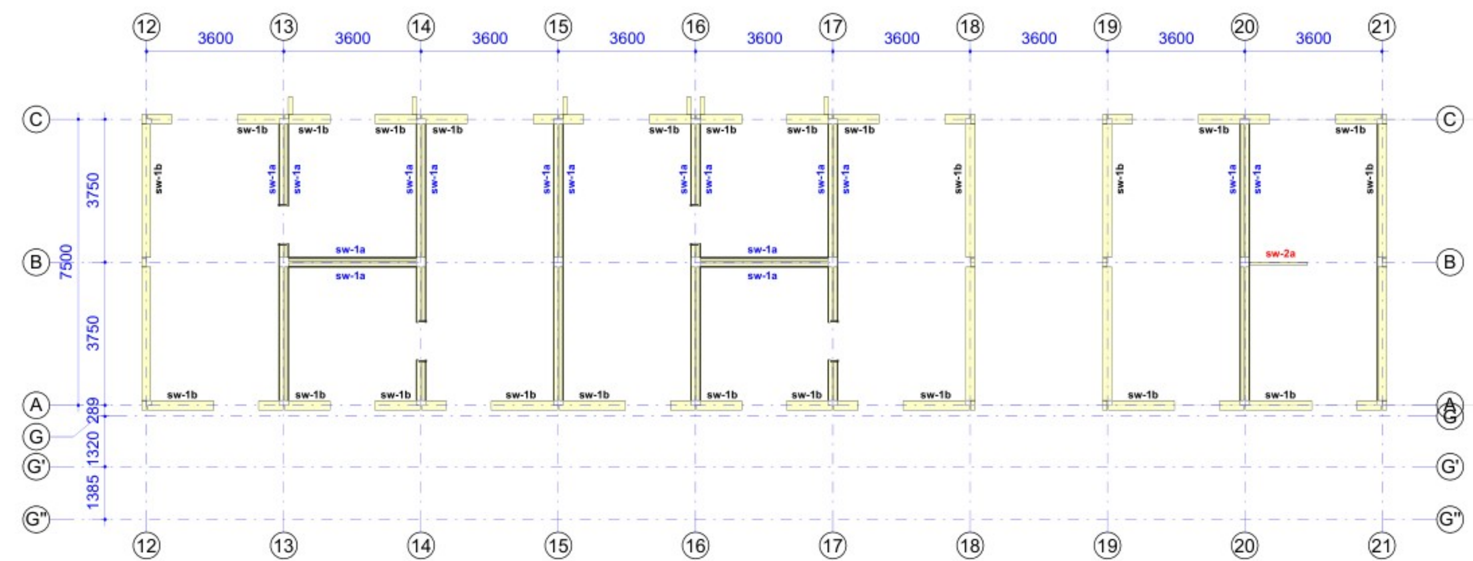
overzicht stabiliteitswanden type sw-1a = 38x89 h.o.h. 610 / sw-1b = 38x235 h.o.h. 610 / sw-2a = 38x89 h.o.h. 610
