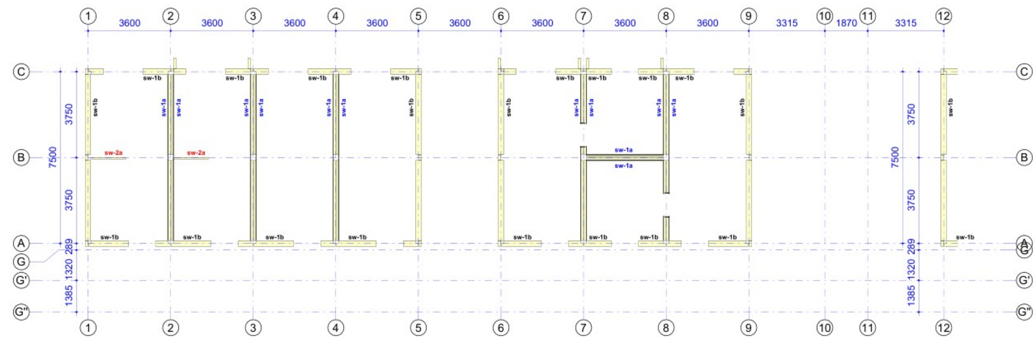
overzicht stabiliteitswanden
