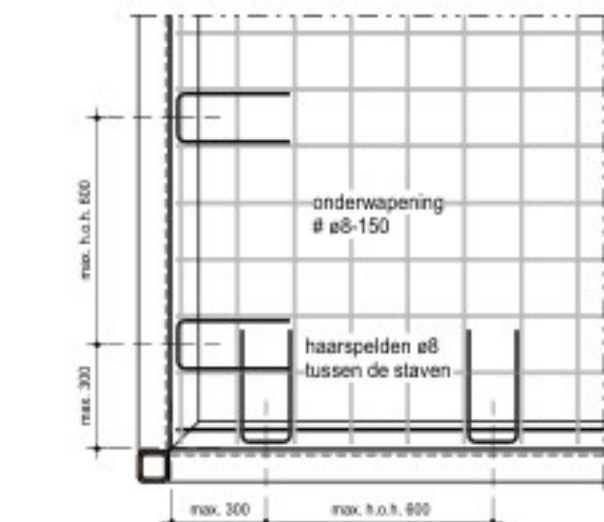
principe plaatsing van de haarspelden bij onderwapening t.p.v. bovenwapening zijn geen haarspelden nodig.
