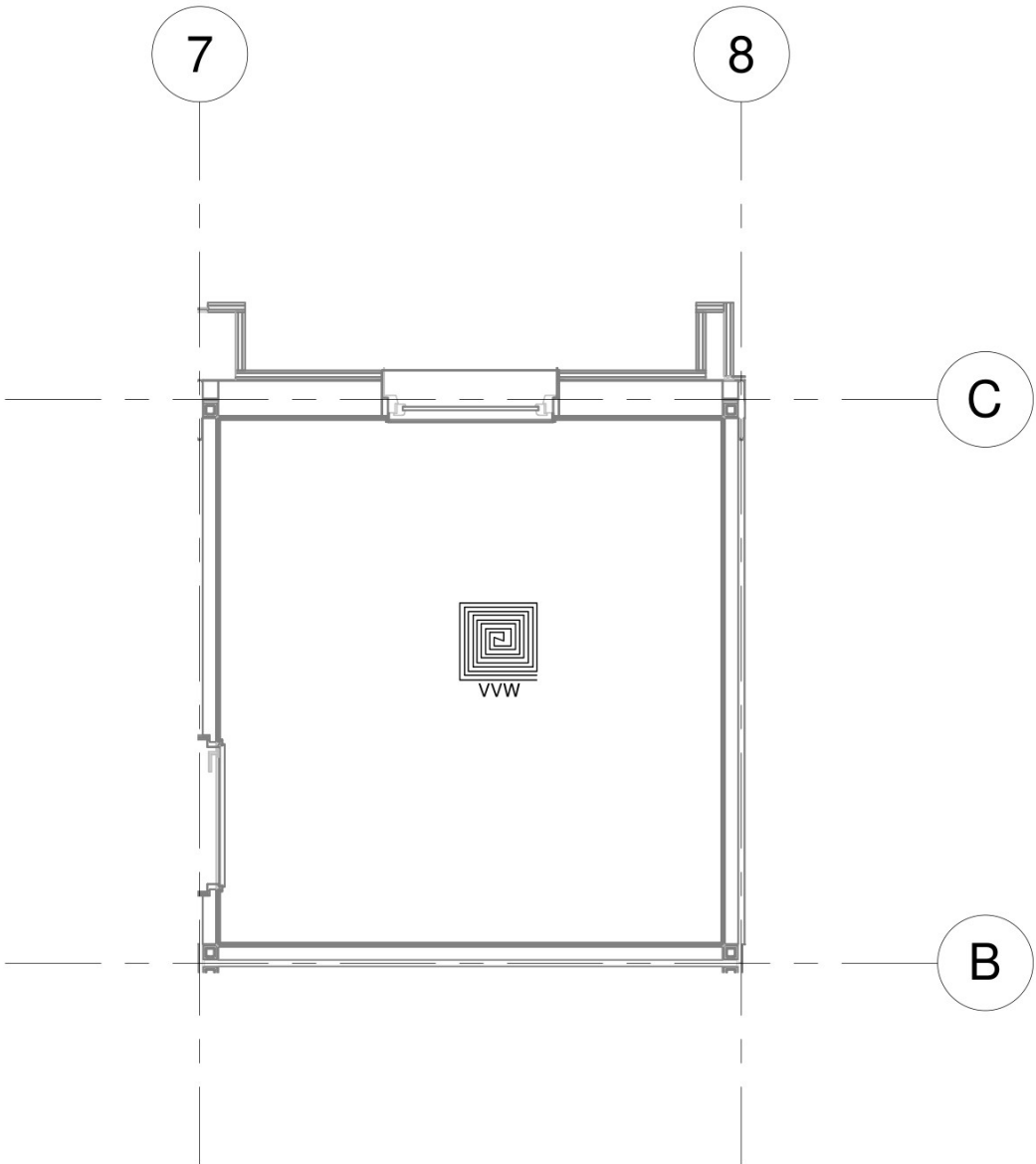
1 V00 - W56_Leidingen_Klimaat - BW-01L-2 1 : 50
