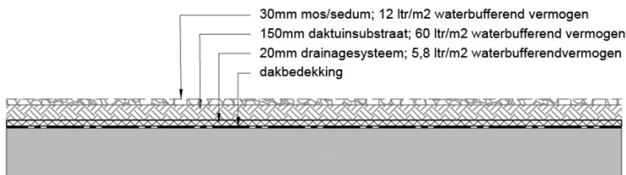
Principe profiel, mos/sedumdak Schaal 1:20
