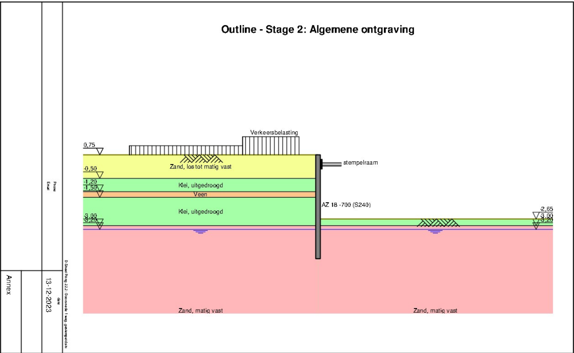
Berekeningsinvoer D-Sheet Piling, gestempelde damwand, weg stage 2
