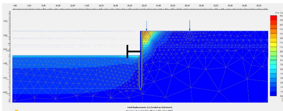
verplaatsingen ondergrond stage 6 - afstempelen keldervloer
