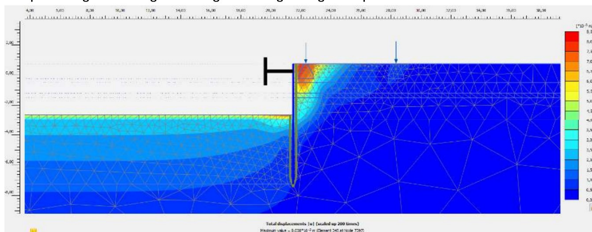
verplaatsingen ondergrond stage 5 - algemene ontgraving
