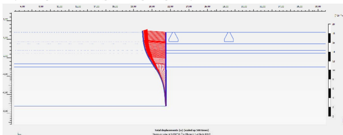
verplaatsing damwand stage 5 - algemene ontgraving
