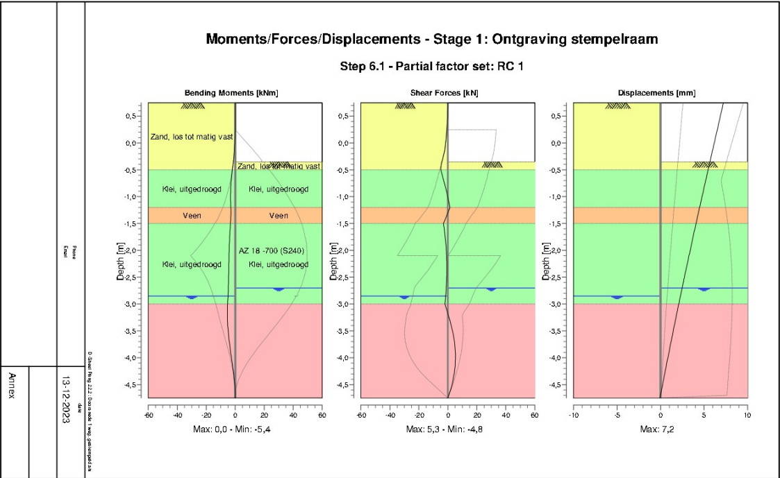
Berekeningsresultaat D-Sheet Piling, gestempelde damwand, weg stage 1, UGT
